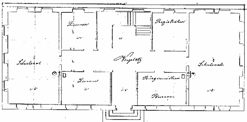
Grundriß des 1. Stockwerkes.
