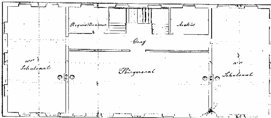
Grundriß des 1. Stockwerkes.
